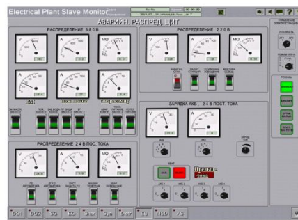
ГРЩ СЭЭС ERS 4000 (5000) - RO-RO
