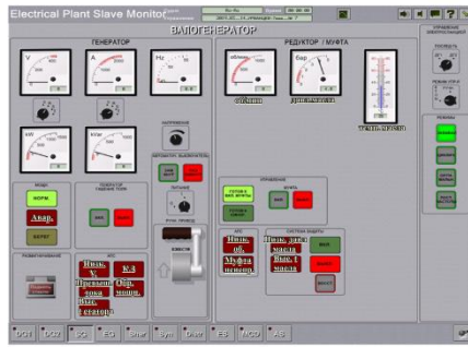
ГРЩ СЭЭС ERS 4000 (5000) - RO-RO
