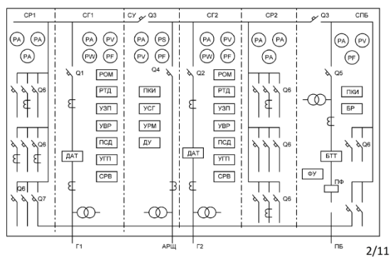
ГРЩ СЭЭС ERS 4000 (5000) - RO-RO
