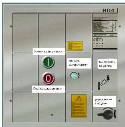
Высоковольтный автоматический выключатель
