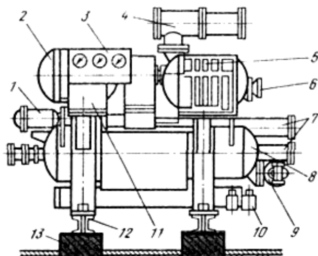
Рисунок 1 – Общий вид винтового компрессора на фундаменте
